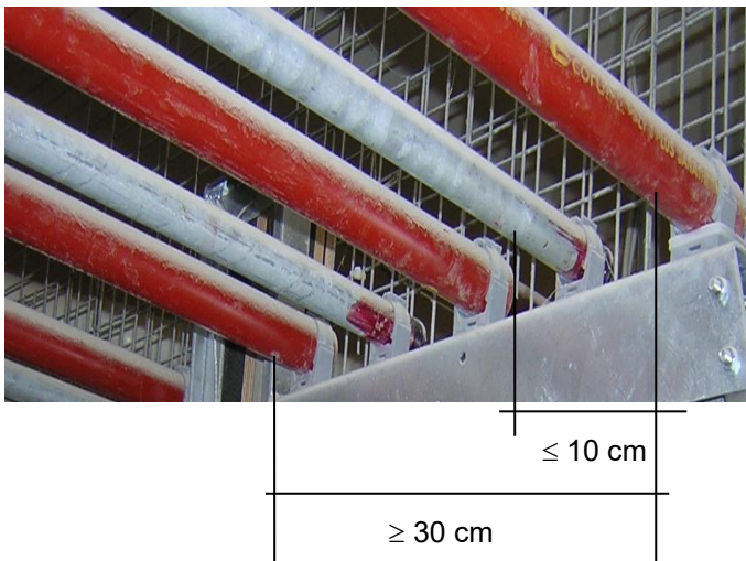
Fig. 5a Caillebotis en tubes métalliques
