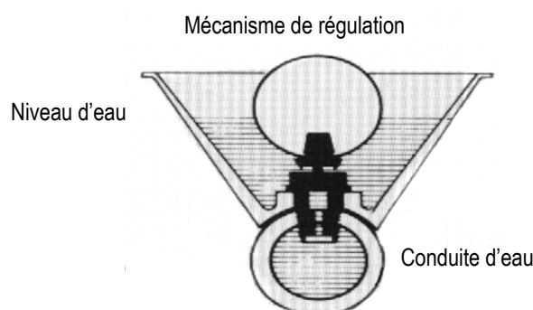
Fig. 3 Coupe transversale d'un abreuvoir à godets
