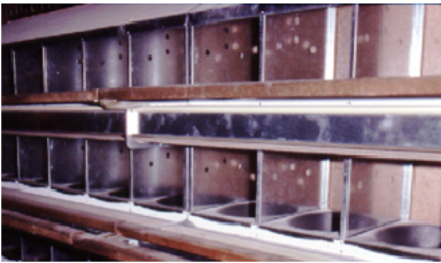
Fig. 6a Nids individuels avec des coques en matière synthétique
